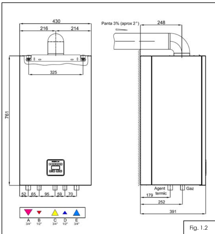
Fig. 1.2 Dimensiuni de gabarit si pozitii de montaj
